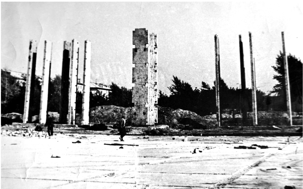
Ил. 8. Возведение каркаса пилонов [Архив МАУК «Музей Новосибирска»] Fg. 8. Erection of the frame of the pylons [Museum of Novosibirsk]
