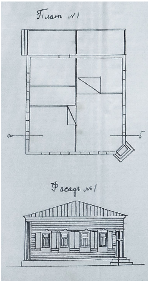
Ил. 2. План дома
